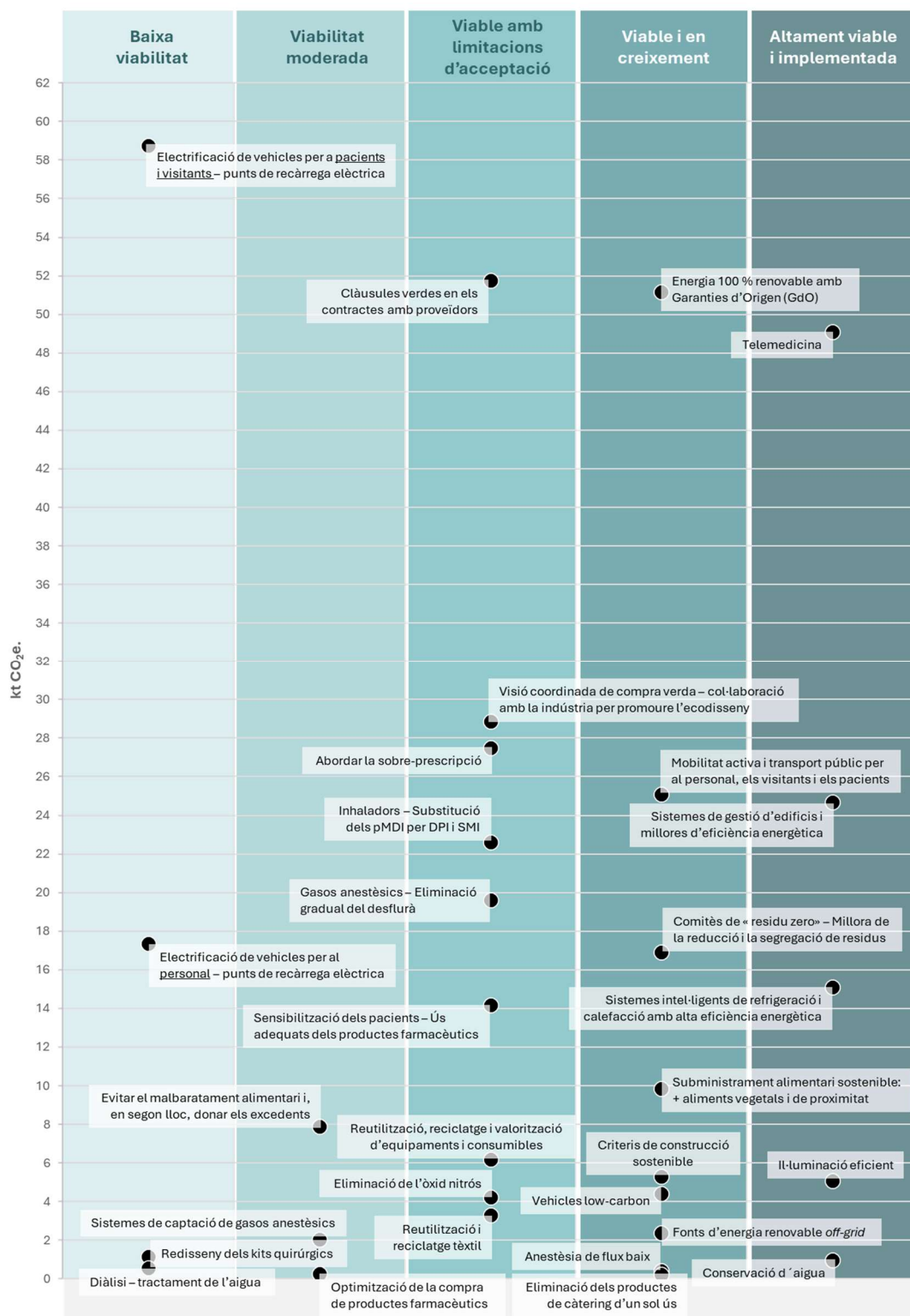
Figura 10. Potencial de reducció de la petjada de carboni i nivells de viabilitat de les mesures de mitigació.
