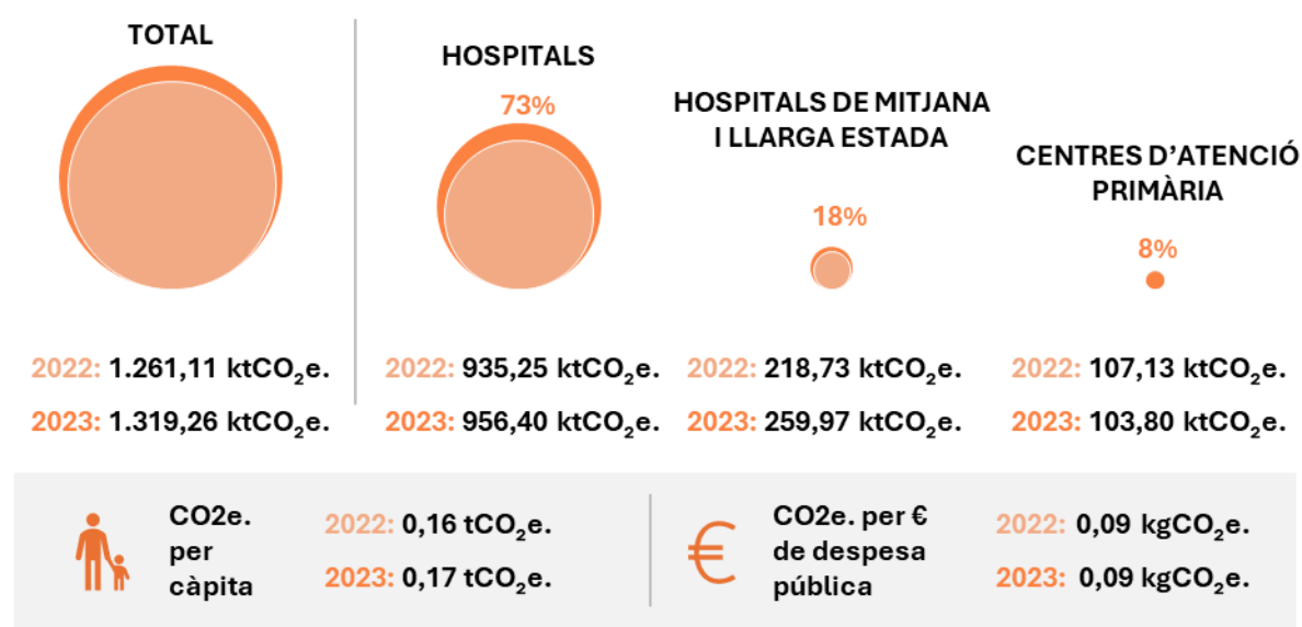
Figura 5. Petjada de carboni 2022-2023.
